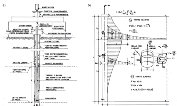
Figura 6. a) Prove di trazione su tiranti eseguibili anche durante le indagini geognostiche oltre che preliminari di cantiere; b) Stato tensionale per scorrimento fra cilindri concentrici.
