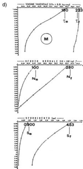
Figura 7. Analisi a ritroso, dal tiro N e dallo spostamento s, delle tensioni tangenziali \tau di aderenza agli stati limite di esercizio (SLE) e ultimo (SLU) che diventano circa uniformi in argille marnose (M).
