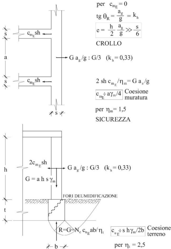
Figura 1. Ruolo antisismico della coesione nelle costruzioni in muratura (STR), consistenti ben ammassate o presidiate da ricorsi di mattoni o catene e con solai lignei o tessuti paralleli, caratteristiche di tanti borghi italiani plurisecolari, e ruolo della coesione non drenata nel caso di terreno consistente di fondazione (GEO).
