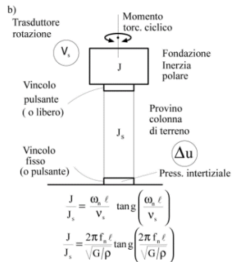
Figura 5. Colonna risonante a torsione.
