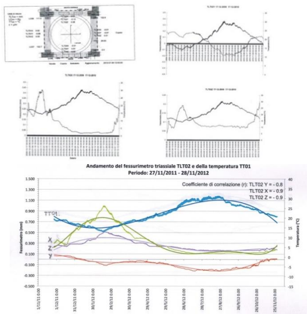
Figura 10. Monitoraggio con trasduttori triassiali TL02-XYZ nella chiave dell'arcone, lato navata centrale, crollata in parte davanti all'altare: confronto con le oscillazioni termiche annuali TT01 prima del consolidamento con deriva verticale 0,2 mm su 0,4 mm della lesione centinata e azzerata dopo il consolidamento con il ricentraggio dei carichi della cupola, togliendole l'eccentricità sui piloni.
